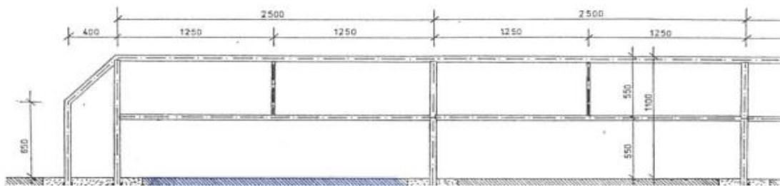
Obrázek 4 – Schéma silničního (dopravně bezpečnostního) zábradlí s výplňovým prutem bez vodící funkce pro nevidomé a slabozraké
