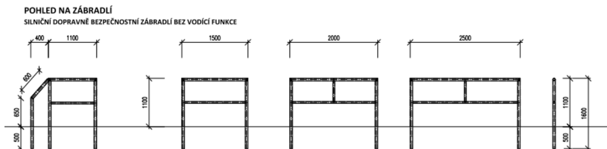
Obrázek 5 – Schéma silničního (dopravně bezpečnostního) zábradlí s výplňovým prutem a zarážkou pro slepeckou hůl
